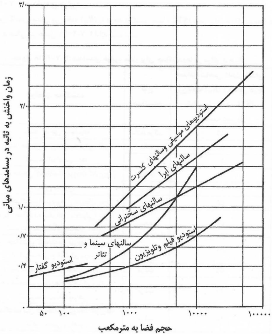
شکل ۱۸-۲-۷-۱: نمودار زمان واخشی بهینه در فضاهای مختلف
